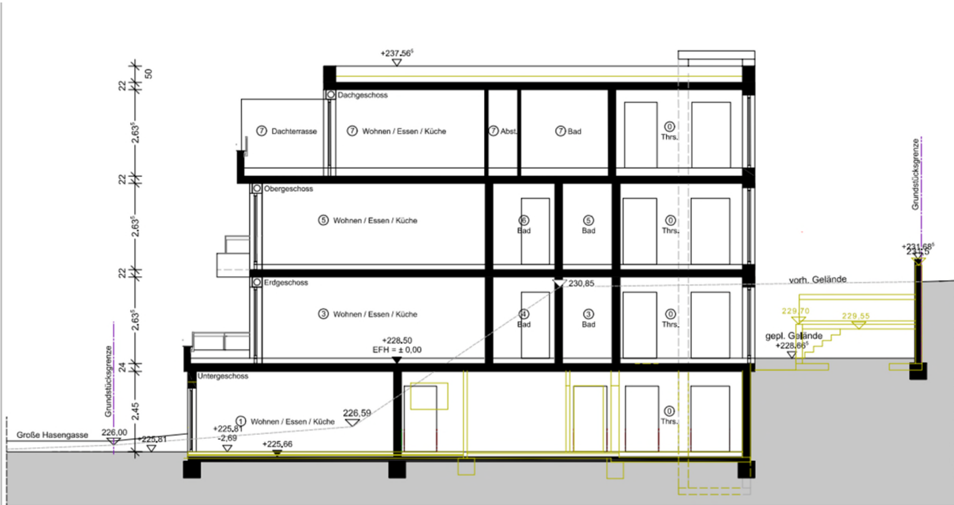
Schnitt A-A
