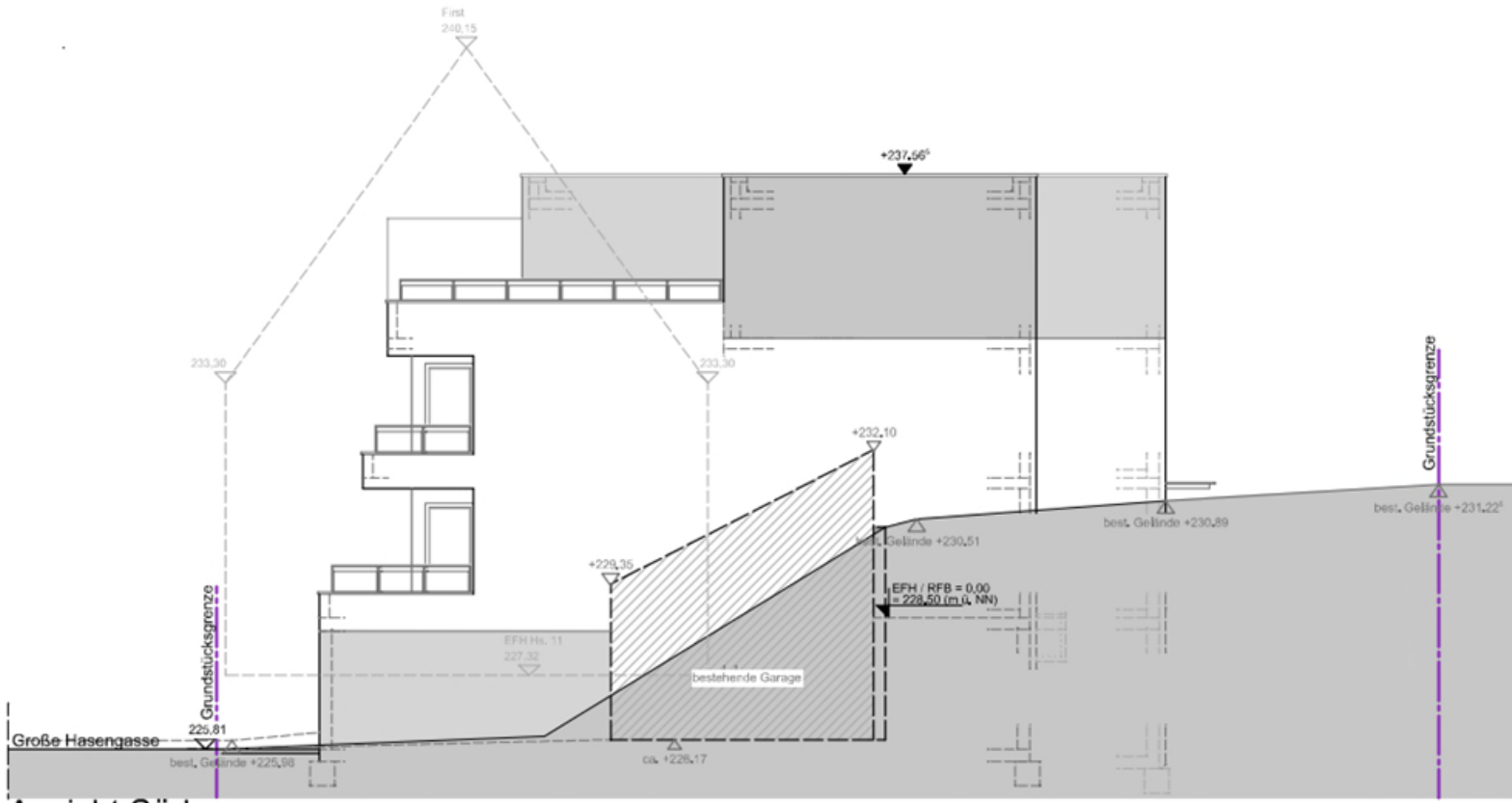
Ansicht Süd
