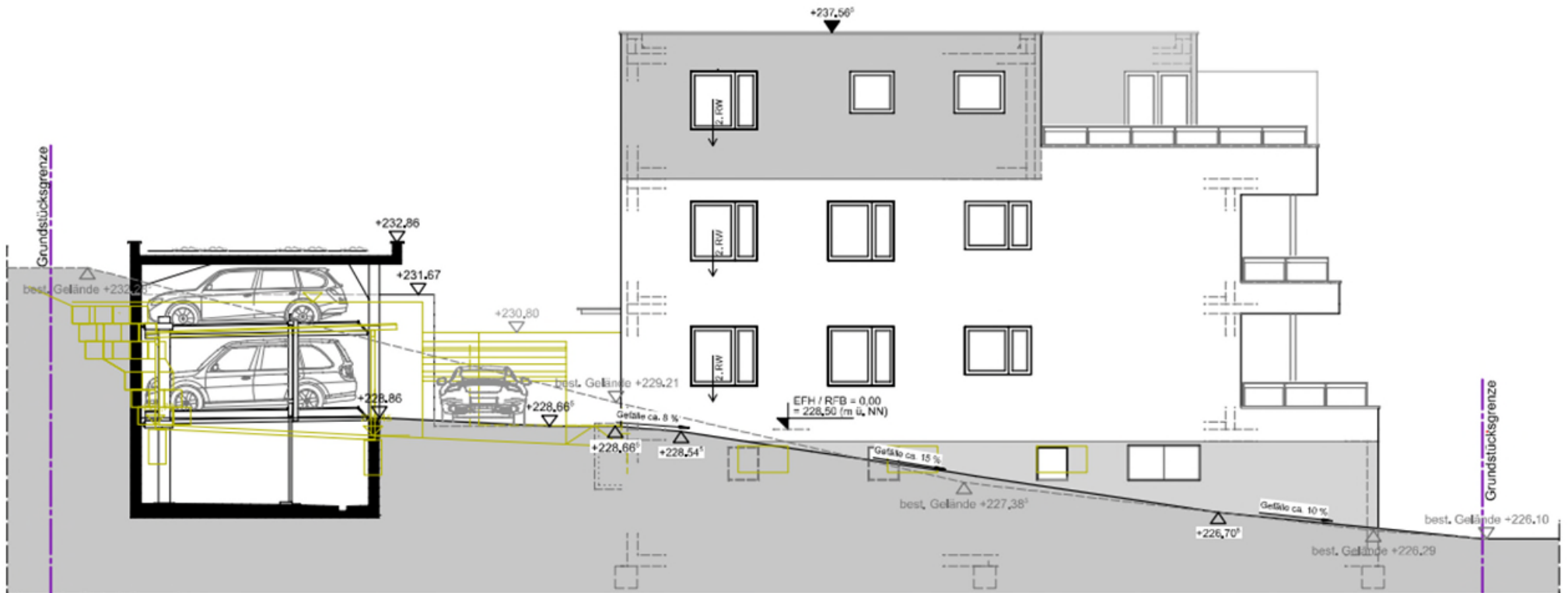
Ansicht Nord
